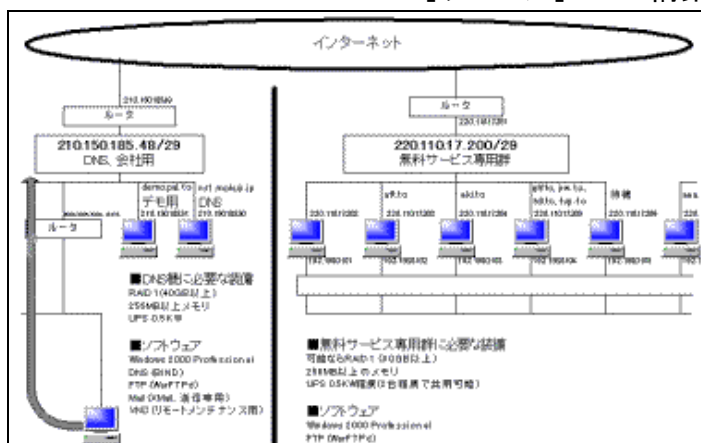
[サンプル] WAN 構築
