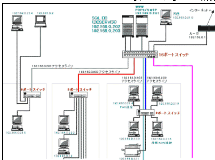
[サンプル] LAN 構築
